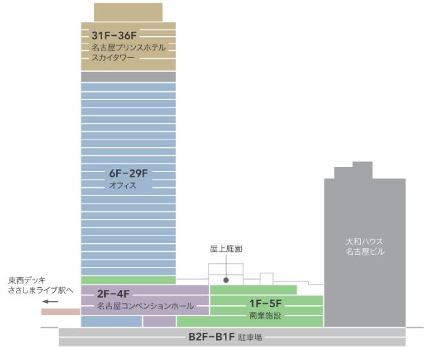
フロア構成
